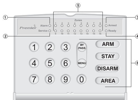
Premier RKP4/8/16
